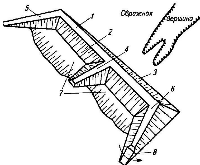
Рисунок 2 - Общий вид водозадерживающего вала:
