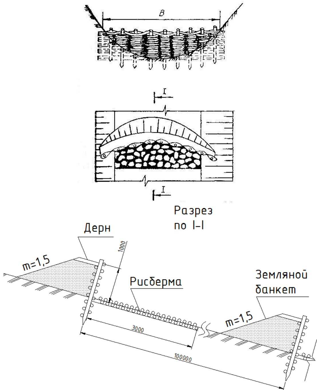
Рисунок 7 - Плетневая запруда с земляным банкетом.
