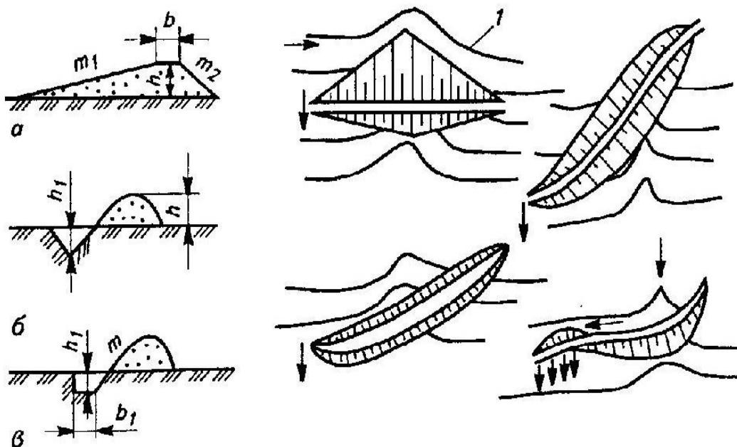
Рисунок 1 - Распылители стока (а) и валы-канавы (б, в) в разрезе (слева) и в плане (справа): 1 – горизонталь поверхности.
