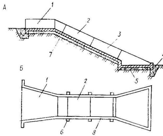
Рисунок 6 - Схема быстротока: А – продольный разрез; Б – план; 1 – водоприемник; 2 – лоток; 3 – водовыпуск; 4 – глиняный замок; 5 – щебень; 6 – упорный брус; 7 – основание сооружения; 8 – стенки сооружения.
