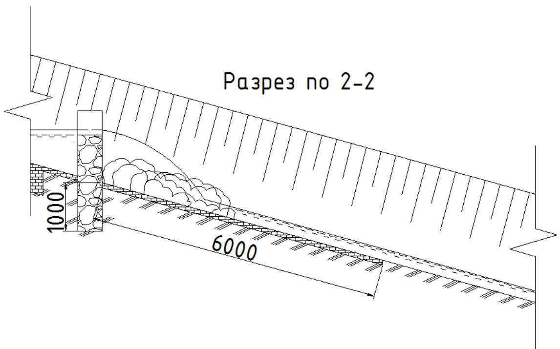
Рисунок 8 - Каменная запруда
