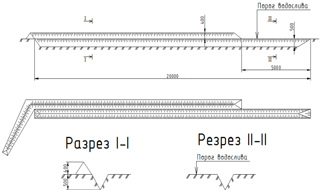
Рисунок 3 - Распылитель стока.
