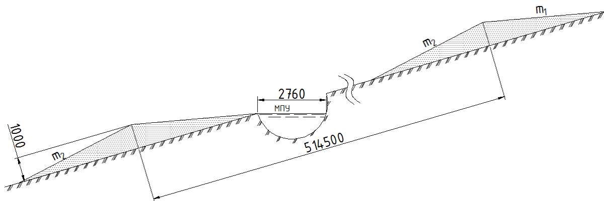
Рисунок 5 - Валы с широким основанием:
