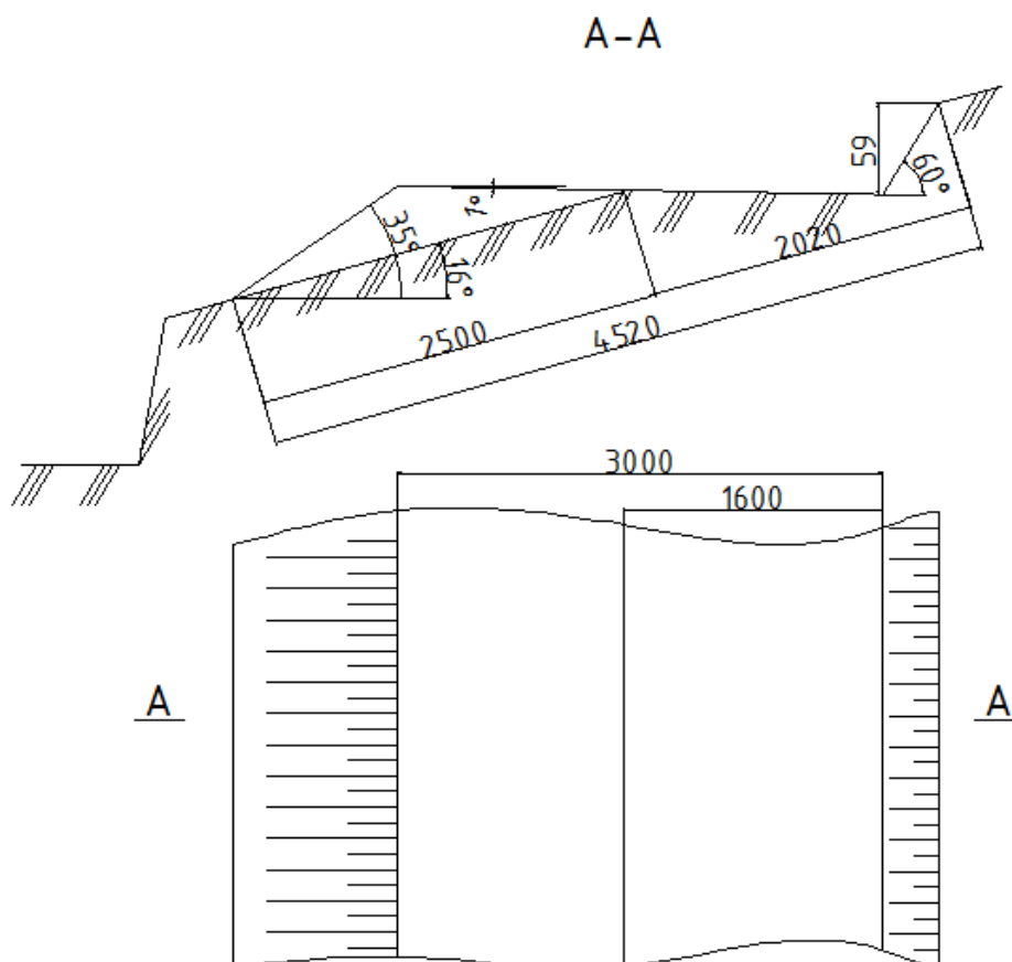
Рисунок 4 - Схема террасы
