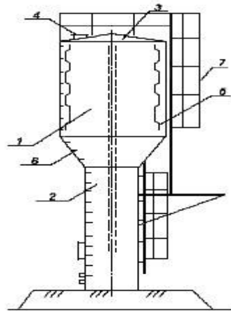
Рисунок 10 Водонапорная башня
