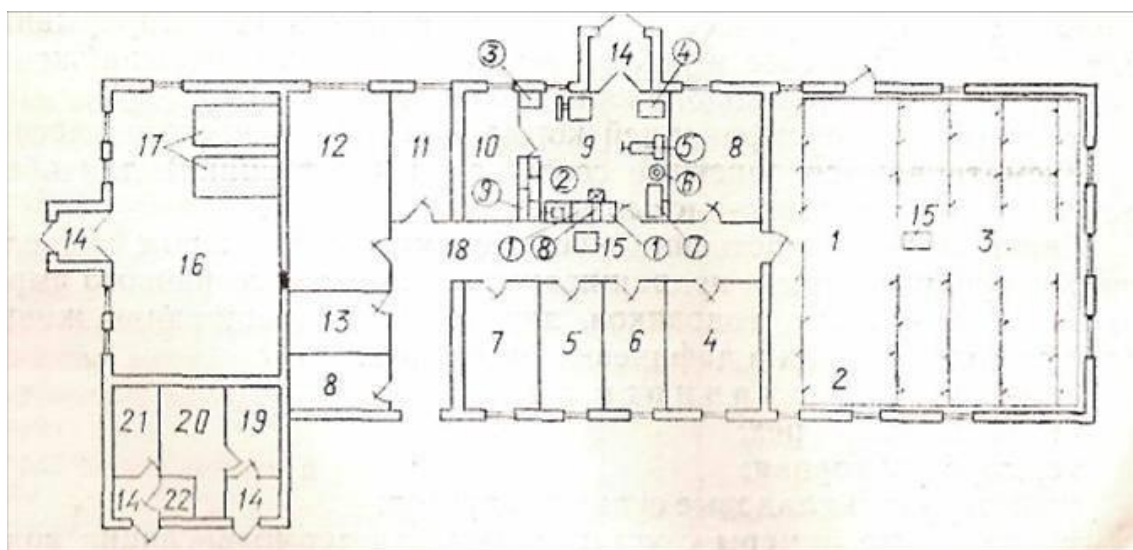
Рис.1. Схема лососевого завода
